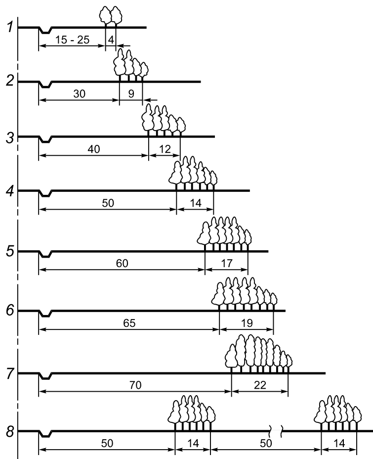
Объемы снегоприноса: 1 — 25 м³/м; 2 — 50 м³/м; 3 — 75 м³/м; 4 — 100 м³/м; 5 — 125 м³/м; 6 — 150 м³/м; 7 — 200 м³/м; 8 — 250 м³/м
